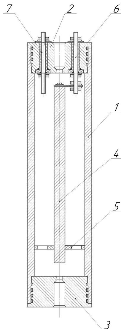
Рис. 2. Чертеж измерительной ячейки.
