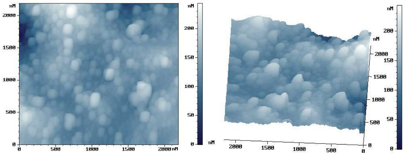
Рисунок 4.23 – 2D (слева) и 3D (справа) изображения АСМ исследовании рельефа на поверхности силицида платины в периферийной области (низкоинтенсивной) пятна облучения ArF-лазером ( \lambda = 193 нм, 20 импульсов; 4.5 \text{ Дж/см}^2 , частота 10 Гц)
