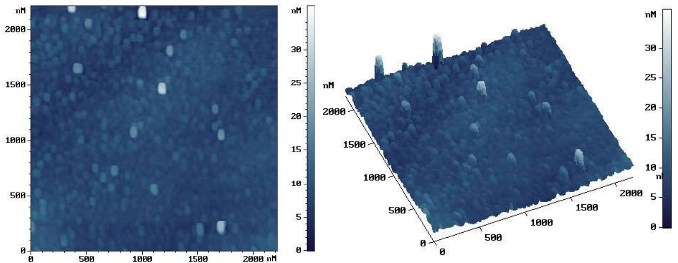
Рисунок 4.20 – 2D (слева) и 3D (справа) изображения АСМ исследования рельефа на поверхности нитрида кремния в периферийной области (за пределами зоны лазерного расплава) пятна облучения ArF-лазером ( \lambda = 193 нм, 20 импульсов; 4.5 \text{ Дж/см}^2 , частота 10 Гц).
