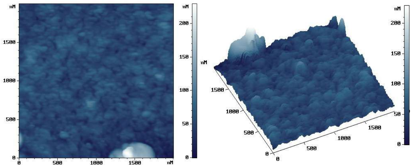
Рисунок 4.24 – 2D (слева) и 3D (справа) изображения АСМ исследовании рельефа исходной необлученной поверхности силицида платины.
