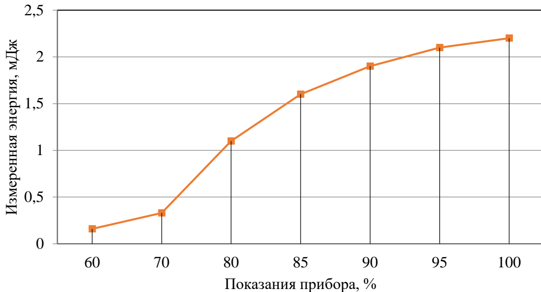
Рисунок 3.15 – Калибровка твердотельного лазера.
