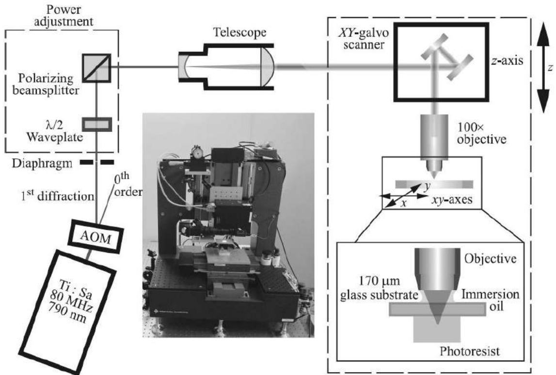
Рисунок 1.11 – Схема и фотография установки 3D-лазерной литографии.
