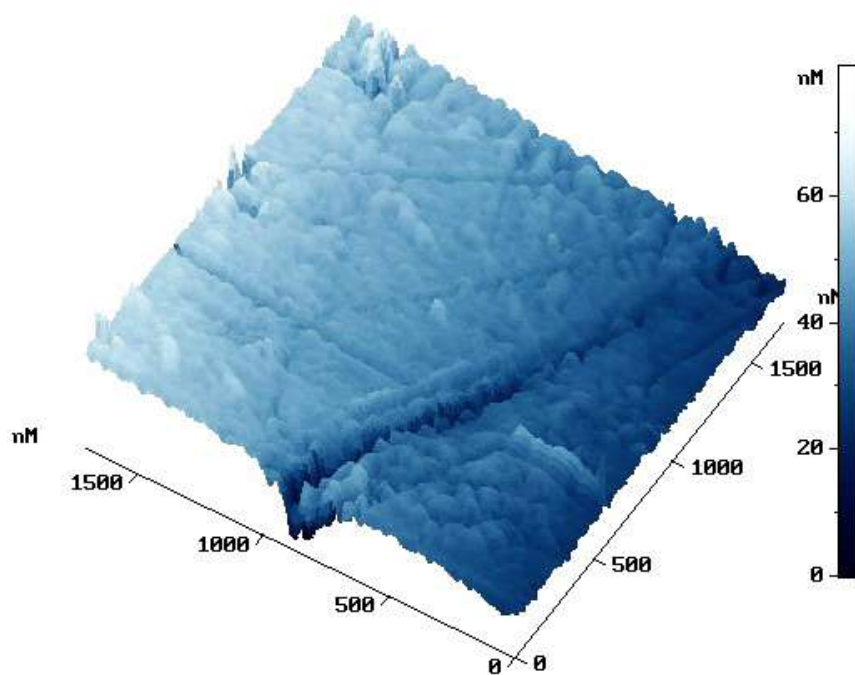
Рисунок 4.11 – 3D изображение АСМ исследования рельефа исходной необлученной поверхности германия.
