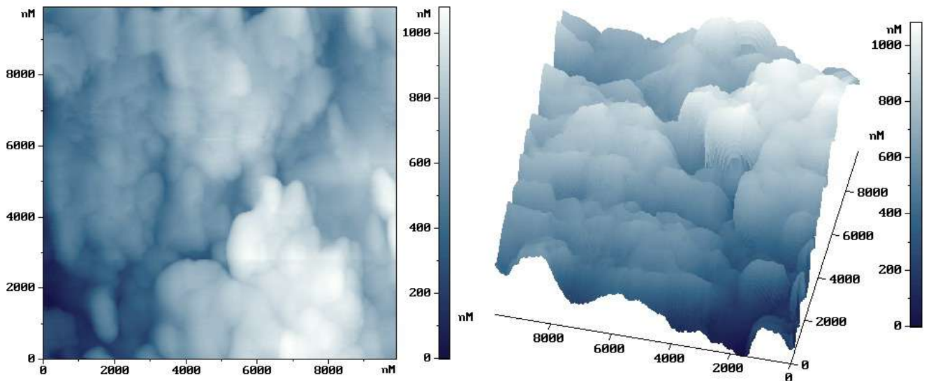
Рисунок 4.26 – 2D (слева) и 3D (справа) изображения АСМ исследования рельефа типа (в) на поверхности титана в периферийной низкоинтенсивной области на краю зоны расплава пятна облучения AgF-лазером ( \lambda=193 нм. 20 импульсов; 5 Дж/см 2 , частота 10 Гц).
