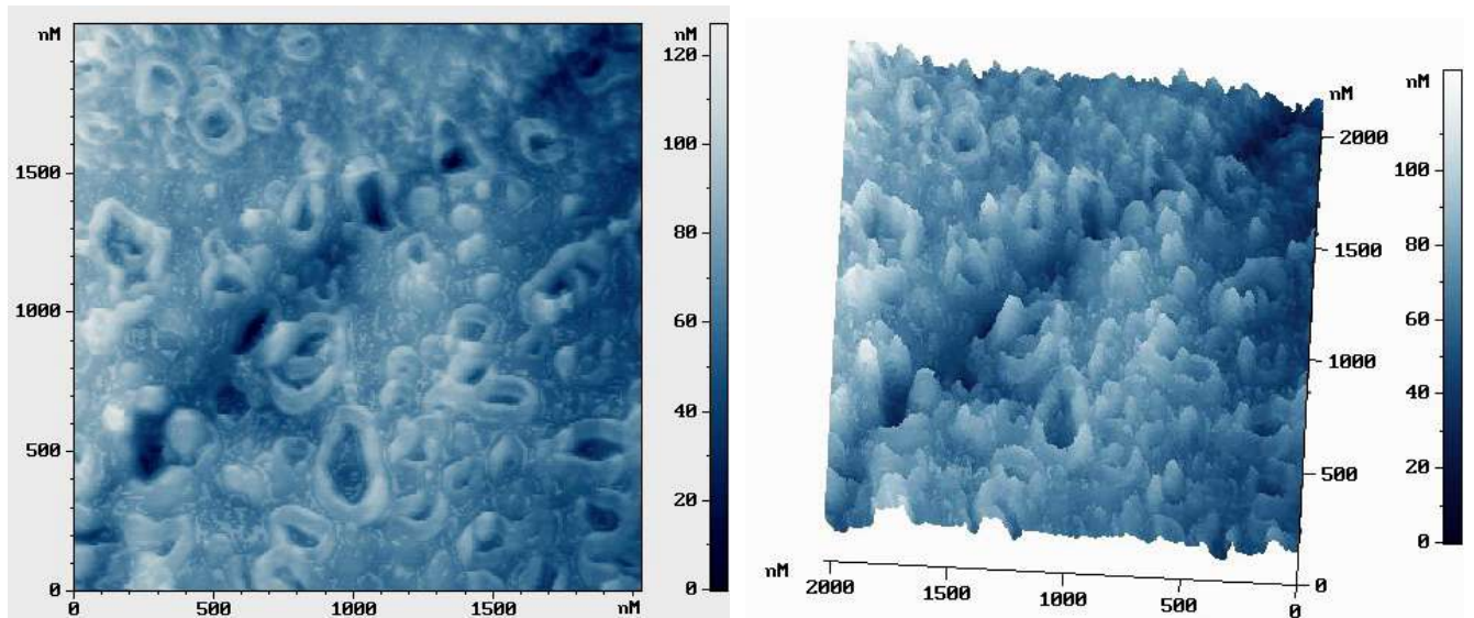
Рисунок 4.13 – 2D (слева) и 3D (справа) изображения АСМ исследования рельефа на поверхности нержавеющей стали в периферийной низкоинтенсивной части пятна облучения AgF-лазером ( \lambda = 193 нм, 20 импульсов; 4 Дж/см 2 , частота 2 Гц).
