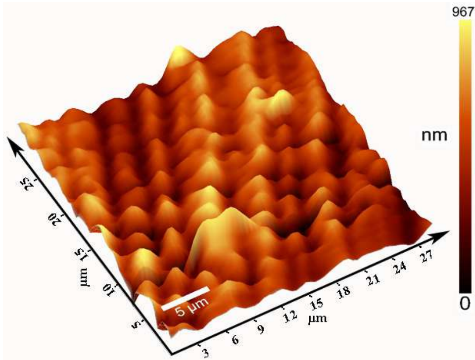
Рисунок 4.34 – 3D изображение АСМ исследования рельефа на поверхности титана в периферийной области пятна облучения лазером на парах меди (700 импульсов; 0,8 мДж; частота 12 кГц)
