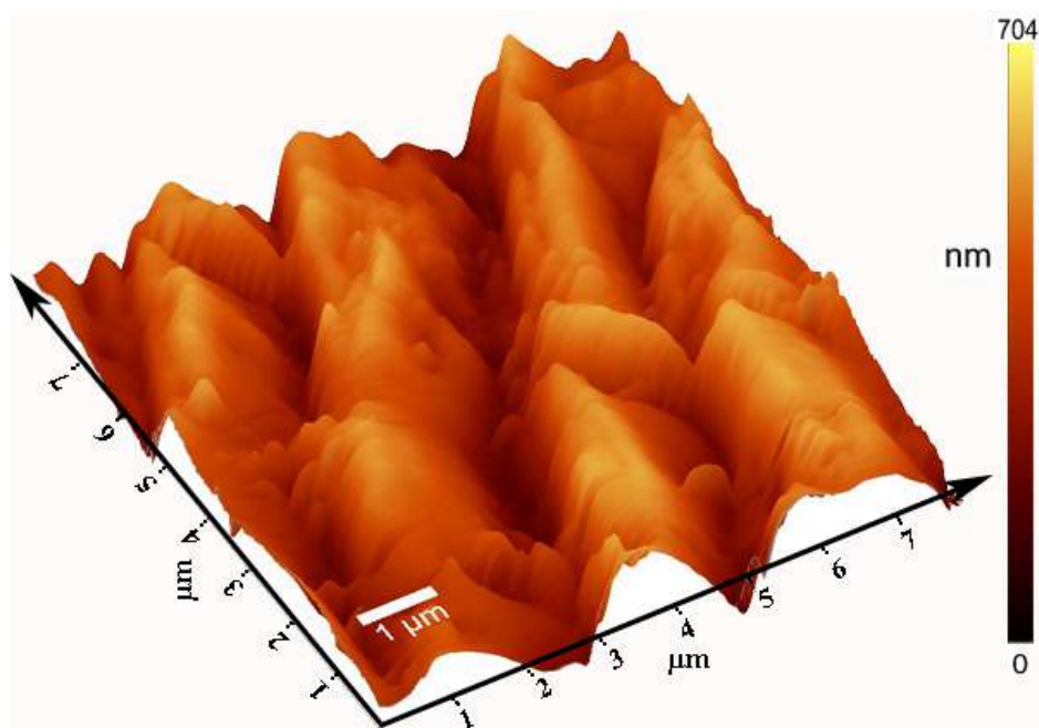
Рисунок 4.33 – 3D изображение АСМ исследования рельефа на поверхности титана в центральной области пятна облучения лазером на парах меди (700 импульсов; 0,8 мДж; частота 12 кГц)
