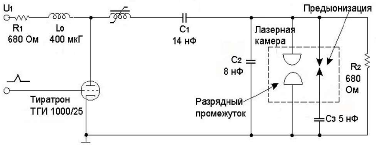
Рисунок 3.6 – Схема накачки лазера.
