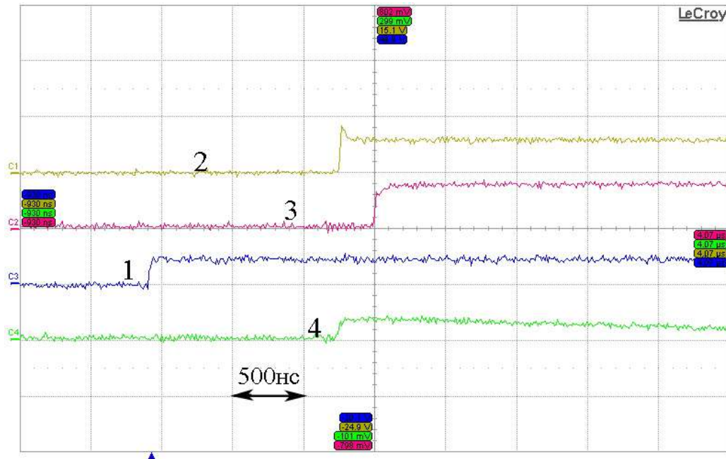
Рисунок. 2.17 – Осциллограмма электрических импульсов синхронизации и импульсов регистрации счетчиком излучения ArF-лазером и Nd:YAG-лазера с задержкой 300 нс. Импульсы 1,2 – синхроимпульсы от генератора ArbStudio 1102, импульсы 3,4 – от счетчика импульсов излучения
