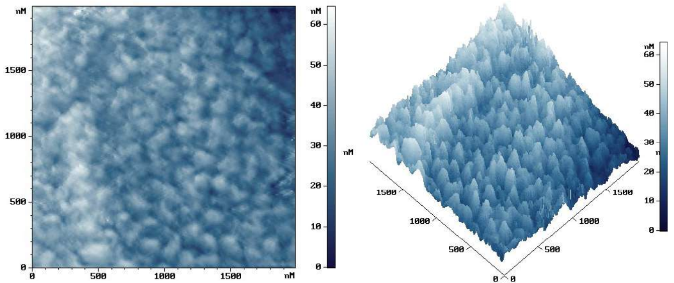
Рисунок 4.17 – 2D (слева) и 3D (справа) изображения АСМ исследования рельефа на поверхности никеля в периферийной области пятна облучения ArF-лазером ( \lambda = 193 нм, 30 импульсов; 5 \text{ Дж/см}^2 , частота 2 Гц)
