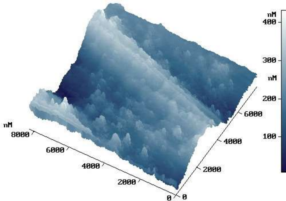
Рисунок 4.18 – 3D изображение рельефа (типа (д) исходной необлученной поверхности никеля.
