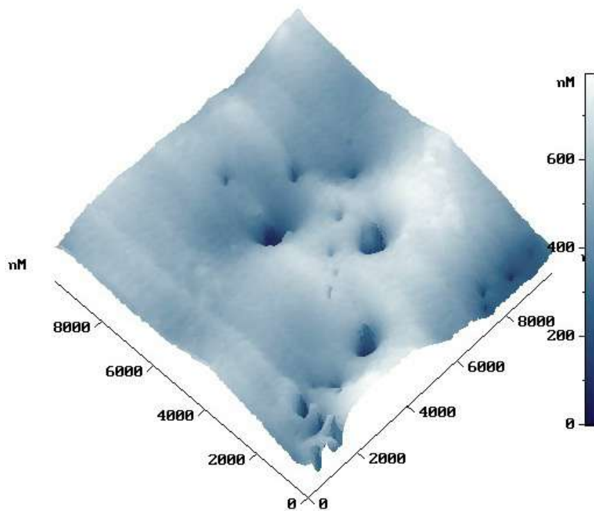
Рисунок 4.15 – 3D изображение АСМ исследования рельефа на поверхности никеля в центральной части пятна облучения ArF-лазером ( \lambda = 193 нм, 30 импульсов; 5 Дж/см 2 , частота 2 Гц).
