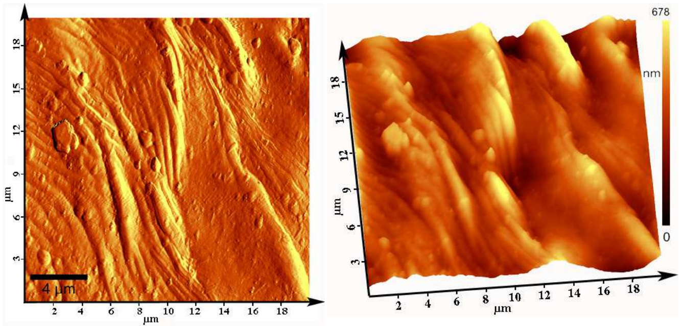
Рисунок 4.30 – 2D (слева) и 3D (справа) изображения АСМ исследования рельефа на поверхности титана в периферийной (на краю зоны расплава) области пятна облучения твердотельным лазером ( \lambda = 355 нм, 30 импульсов; 8.3 Дж/см 2 , частота 10 Гц).
