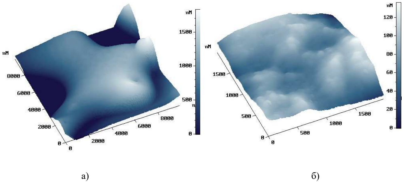
Рисунок 4.22 – 3D изображения с малым (а) и большим (б) увеличением АСМ исследовании рельефа на поверхности силицида платины в центральной части пятна облучения ArF-лазером ( \lambda = 193 нм, 20 импульсов; 4.5 \text{ Дж/см}^2 , частота 10 Гц).
