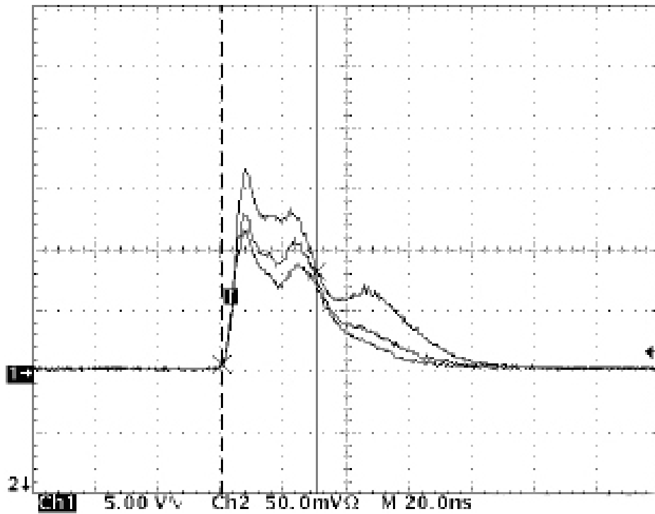
Рисунок 3.7 – Осциллограмма импульсов напряжения на РП (1) и лазерного излучения (2)
