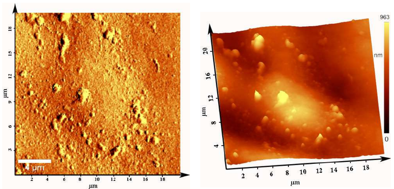
Рисунок 4.29 - 2D (слева) и 3D (справа) изображения АСМ исследования рельефа на поверхности титана в центральной части пятна облучения твердотельным лазером. ( \lambda = 355 нм. 30 импульсов; 8,3 Дж/см 2 , частота 10 Гц).
