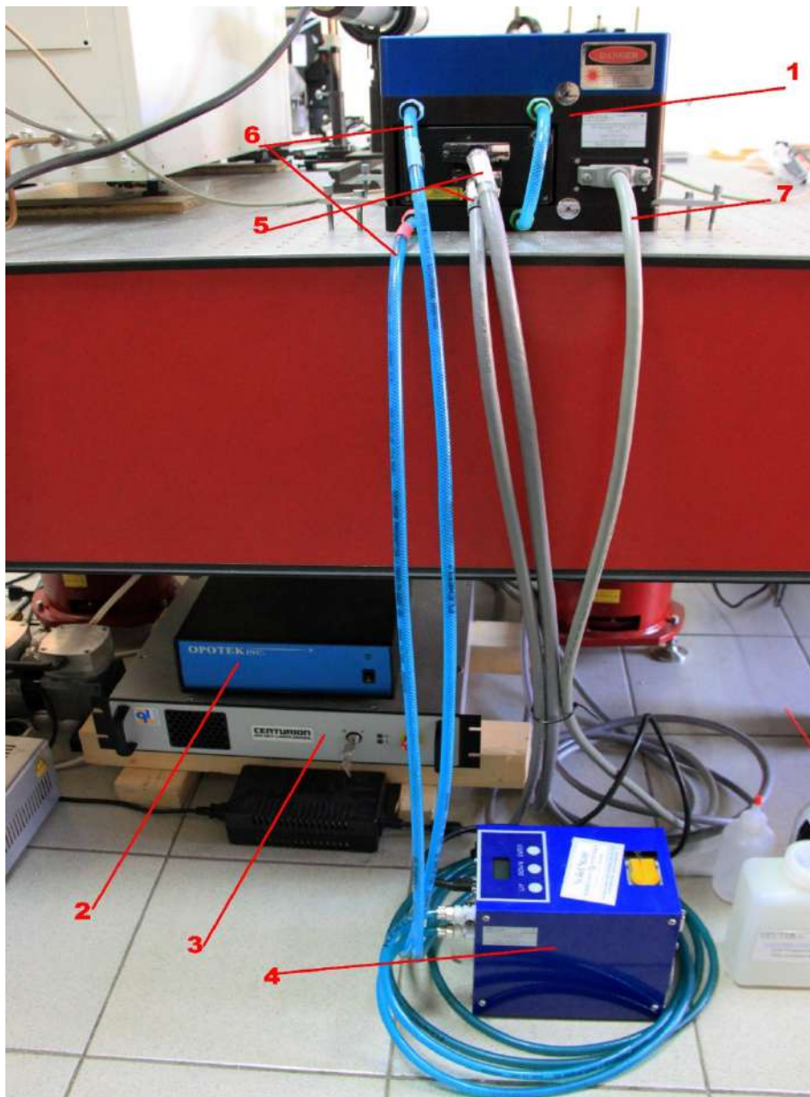
Рисунок 2.9 – Фотография твердотельного лазера HR2731. 1- лазерный модуль, 2- блок управления системой, 3- блок питания, 4- блок охлаждения, 5- силовые кабели подключения блока питания, 6- патрубки подключения охлаждающей жидкости, 7- кабель подключения блока управления.
