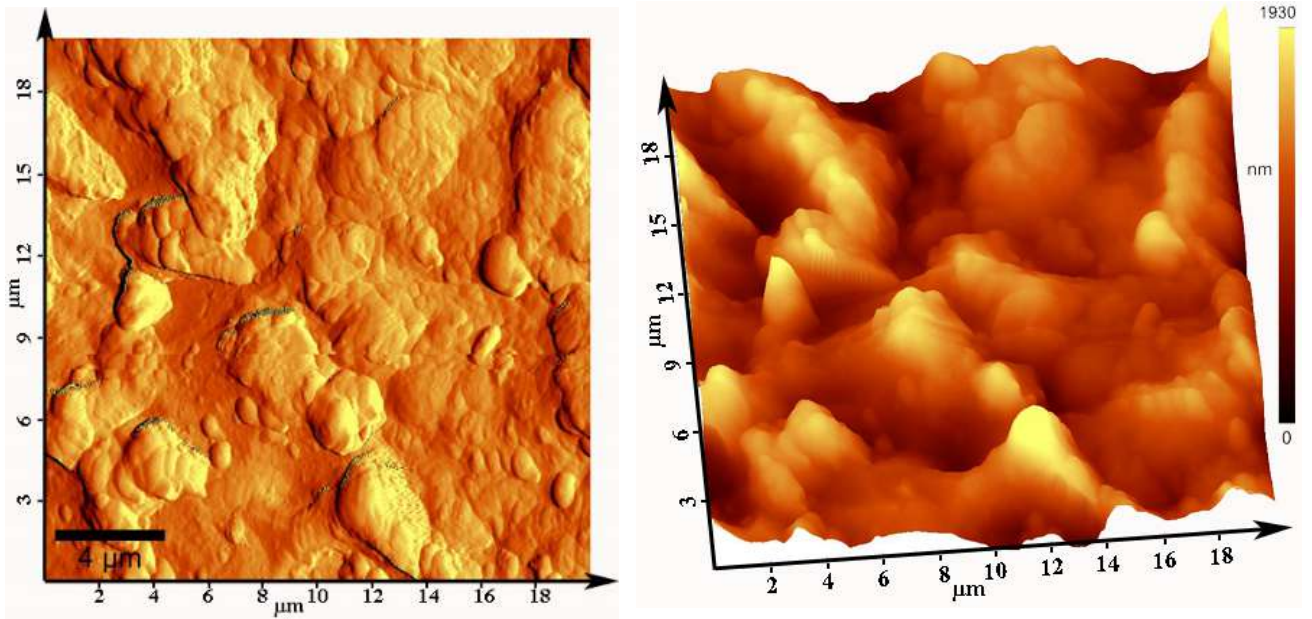
Рисунок 4.32 - 2D (слева) и 3D (справа) изображения АСМ исследования рельефа на поверхности титана на границе пятна облучения твердотельным лазером ( \lambda = 355 нм, 30 импульсов; 8.3 Дж/см 2 , частота 10 Гц).
