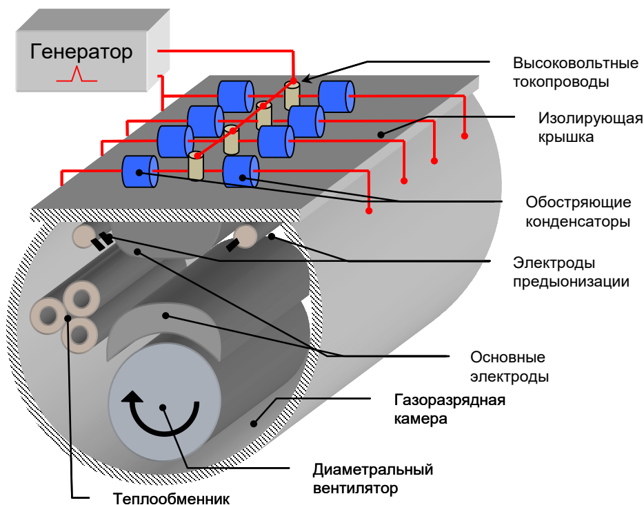
Рисунок 2.8 – Схема металлокерамической газоразрядной камеры.
