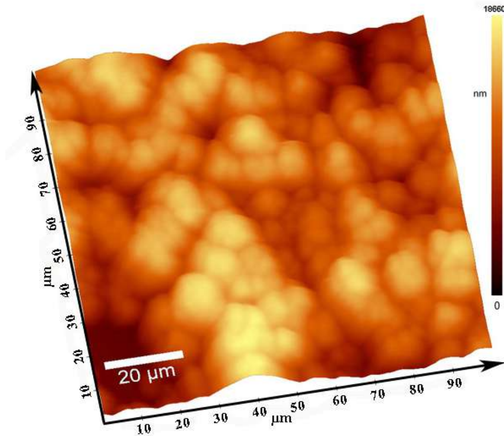
Рисунок 4.40 – 3D изображения АСМ исследования рельефа на поверхности ЭИП из оксида алюминия после облучения сканированием пучка твердотельного лазера ( \lambda = 355 нм, 0,25 мм/с, 1,1 Дж/см 2 , частота 100 Гц).
