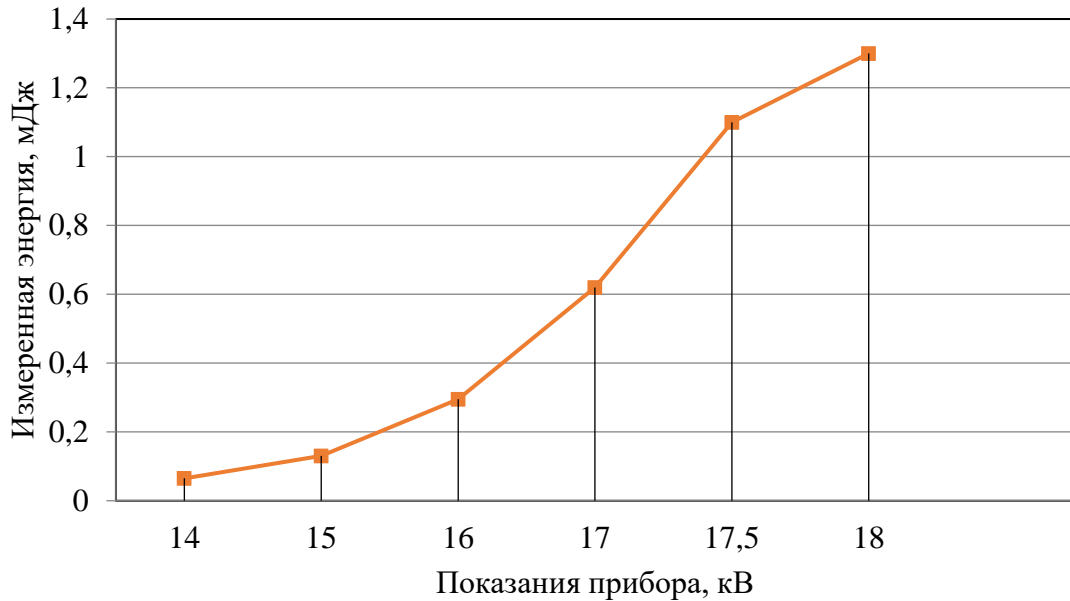
Рисунок 3.14 – Калибровка ArF-лазера.
