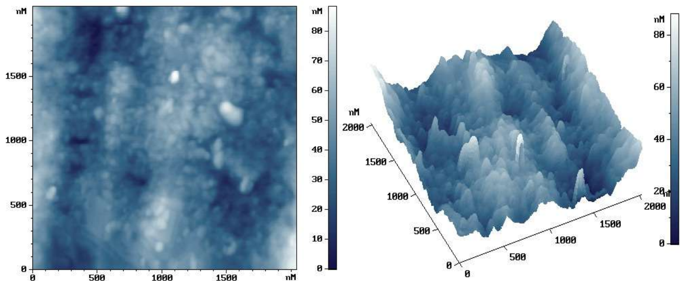
Рисунок 4.28 – 2D (слева) и 3D (справа) изображения АСМ исследовании рельефа исходной необлученной поверхности титана.
