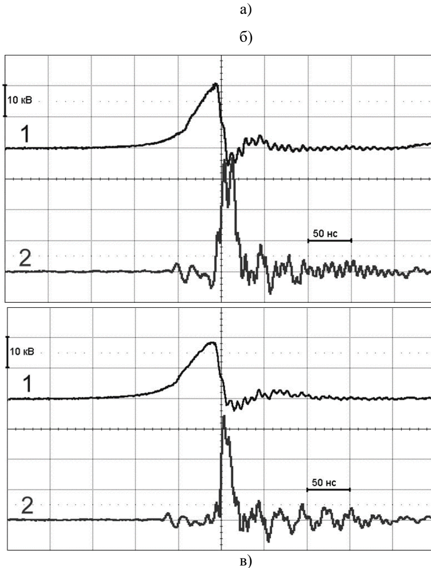
Рисунок 3.3 – Осциллограммы напряжения на РП (2) и генерации излучения 193 нм (1) при разных значениях U_1
