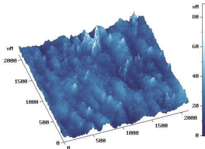
Рисунок 4.14 – 3D АСМ изображение исходной необлученной поверхности нержавеющей стали.
