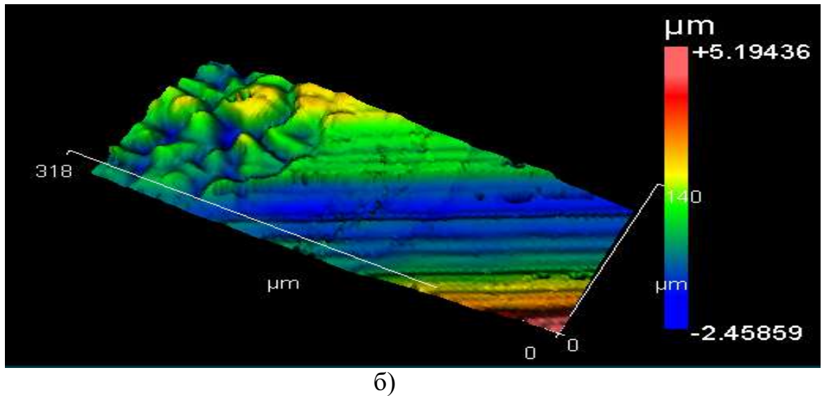
Рисунок 4.6 – а) Фотография поверхности образца стали, сделанная на профилометре. Цифрами 1, 2, 3 обозначены области для измерения на АСМ. б) 3D изображение полученное с помощью профилометрии.
