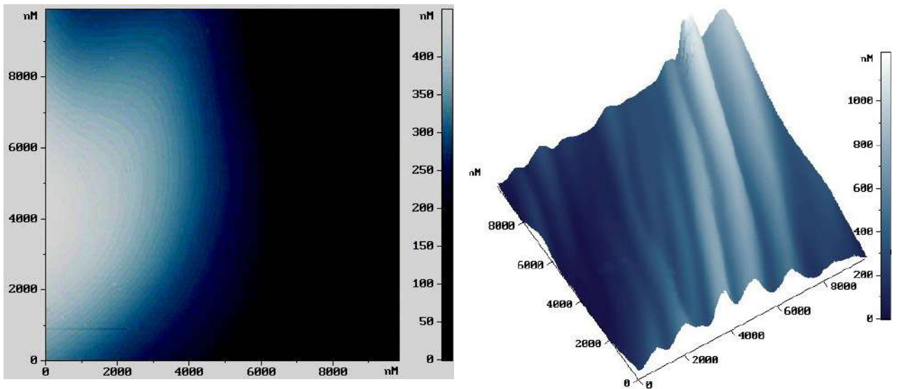
Рисунок 4.8– 2D (слева) и 3D (справа) изображения АСМ исследования рельефа в виде волн на поверхности германия в центральной части пятна облучения AgF-лазером ( \lambda=193 нм. 20 импульсов; 4 Дж/см 2 , частота 2 Гц)
