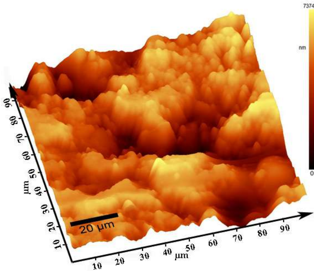
Рисунок 4.41 – 3D изображения АСМ исследовании рельефа на поверхности ЭИП из оксида алюминия после облучения сканированием пучка ArF - лазера ( \lambda= 193 нм, 1 мм/с, 6 Дж/см 2 , частота 100 Гц).
