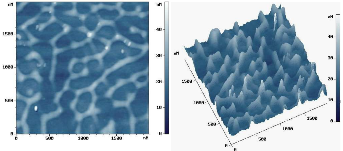
Рисунок 4.9 – 2D (слева) и 3D (справа) изображения АСМ исследовании рельефа на поверхности германия в периферийной низкоинтенсивной области пятна вблизи границы существования расплава ( \lambda = 193 нм, 20 импульсов; 4 Дж/см 2 , частота 2 Гц).
