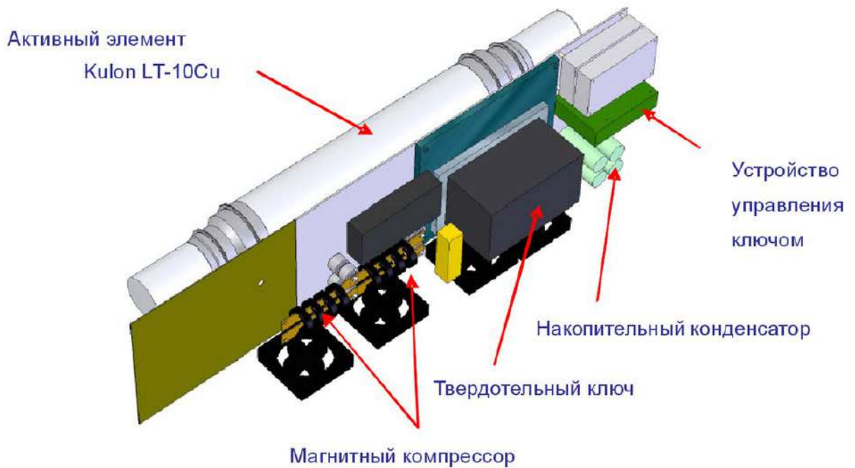
Рисунок 2.4 – Компоновка элементов генератора и активного элемента.
