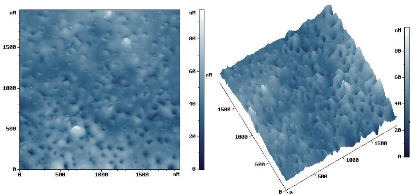
Рисунок 4.12 – 2D (слева) и 3D (справа) изображения АСМ исследования рельефа на поверхности нержавеющей стали в центральной части пятна облучения ArF-лазером ( \lambda = 193 нм, 20 импульсов; 4 Дж/см 2 , частота 2 Гц).
