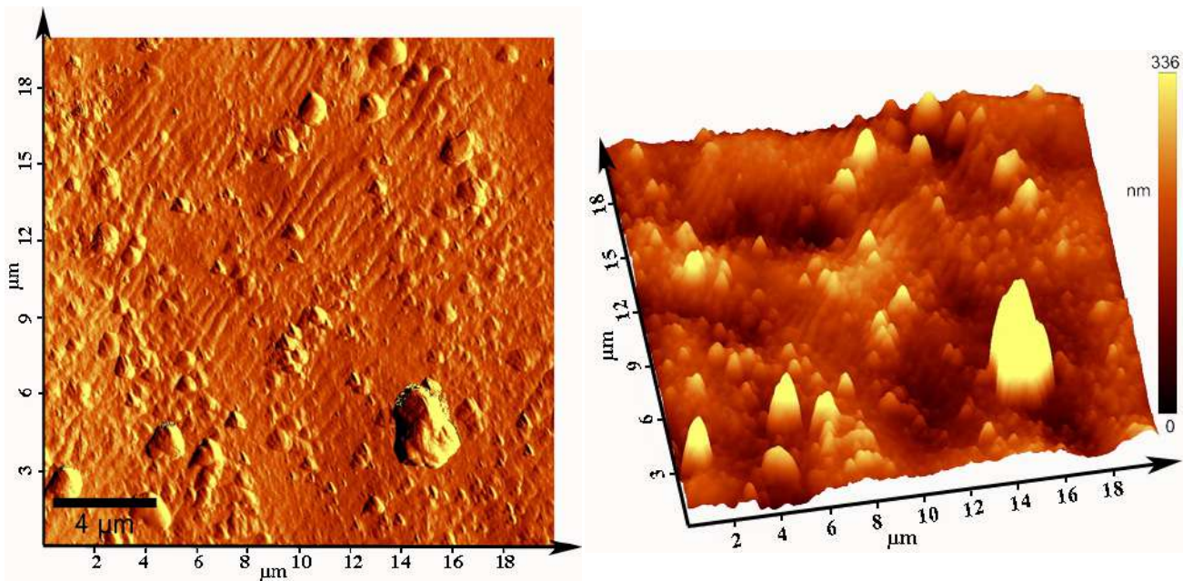
Рисунок 4.31 – 2D (слева) и 3D (справа) изображения АСМ исследования рельефа на поверхности титана в периферийной (за зоной расплава) области пятна облучения твердотельным лазером ( \lambda = 355 нм, 30 импульсов; 8.3 Дж/см 2 , частота 10 Гц).
