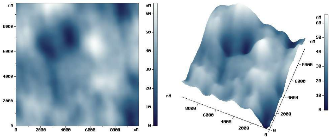
Рисунок 4.25 – 2D (слева) и 3D (справа) изображения АСМ исследования рельефа на поверхности титана в центральной области пятна облучения AgF-лазером ( \lambda=193 нм. 20 импульсов; 5 Дж/см 2 , частота 10 Гц)
