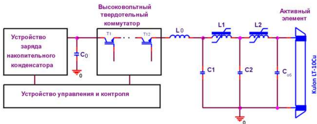
Рисунок 2.5 – Структурная схема лазера на парах меди.
