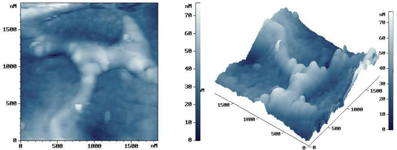
Рисунок 4.16 – 2D (слева) и 3D (справа) изображения АСМ исследования рельефа на поверхности никеля в периферийной области (вблизи границы расплава) пятна облучения ArF-лазером ( \lambda = 193 нм, 30 импульсов; 5 \text{ Дж/см}^2 , частота 2 Гц).
