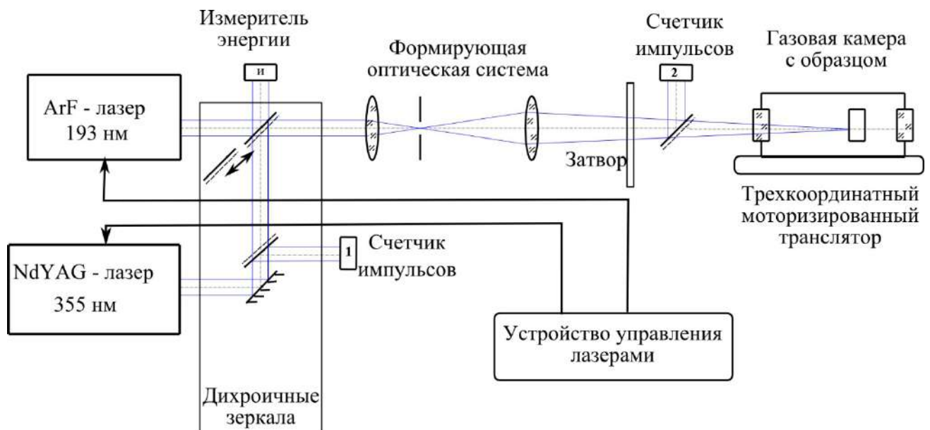
Рисунок. 2.15 – Схема установки для микро- и нано-структурирования с синхронизацией двойных импульсов.
