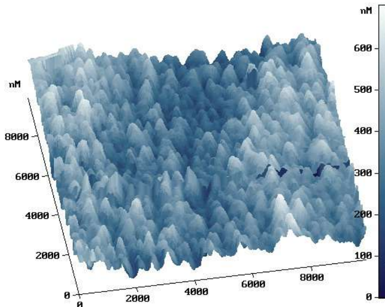
Рисунок 2.2 - Полученные с помощью атомно-силового микроскопа 3D-профили поверхности алмазоподобной пленки после облучения 100 лазерными импульсами с плотностью падающей энергии около 3 \text{ Дж/см}^2 . Видна шероховатость в виде плотно расположенных друг к другу наноструктур – выпуклостей с формой близкой к конусообразной, характерными латеральными размерами 200-600 нм и высоким аспектным отношением (около 1).
