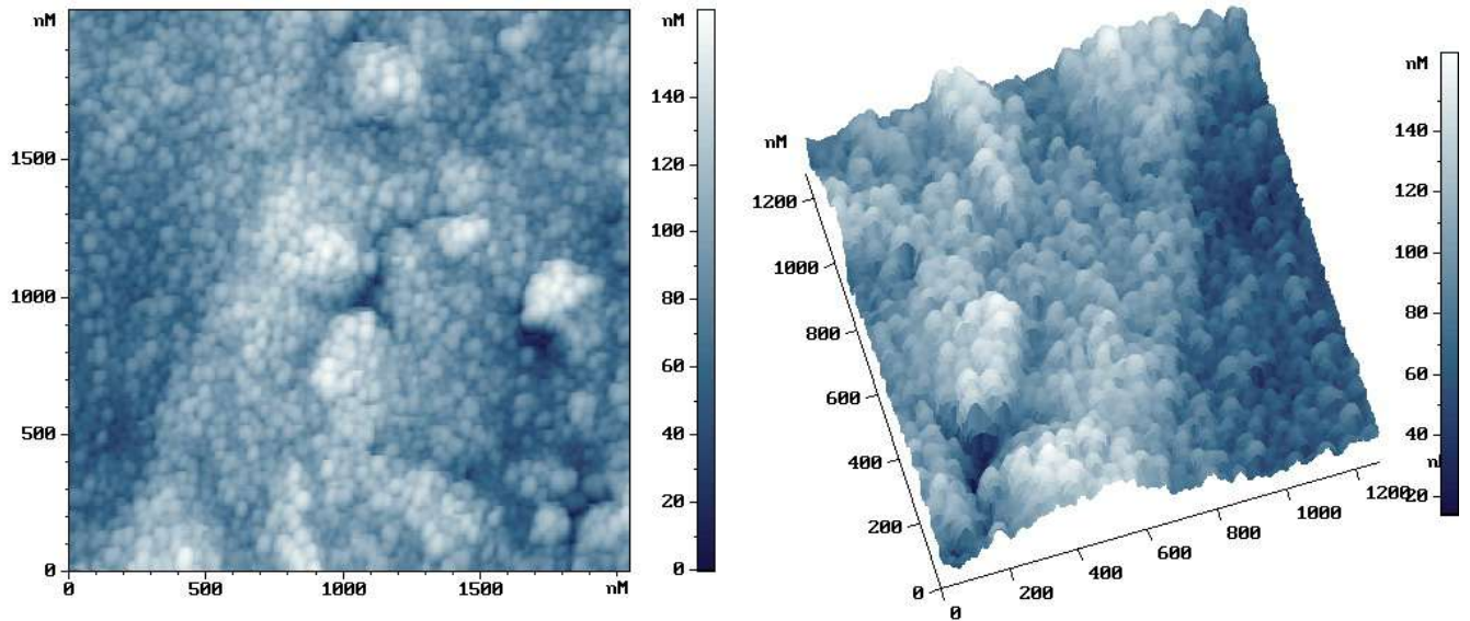
Рисунок 4.27 – 2D (слева) и 3D (справа) изображения АСМ исследовании рельефа типа (г) на поверхности титана в периферийной низкоинтенсивной области пятна облучения ArF-лазером.
