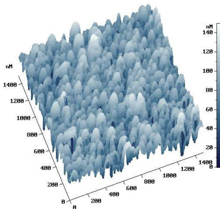
Рисунок 4.10 – 3D изображение АСМ исследования рельефа на поверхности германия в периферийной области пятна ( \lambda=193 нм. 20 импульсов; 4 Дж/см 2 , частота 2 Гц).
