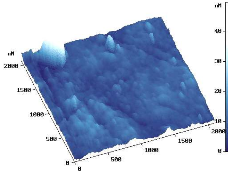
Рисунок 4.21 – 3D изображение рельефа исходной необлученной поверхности нитрида кремния.
