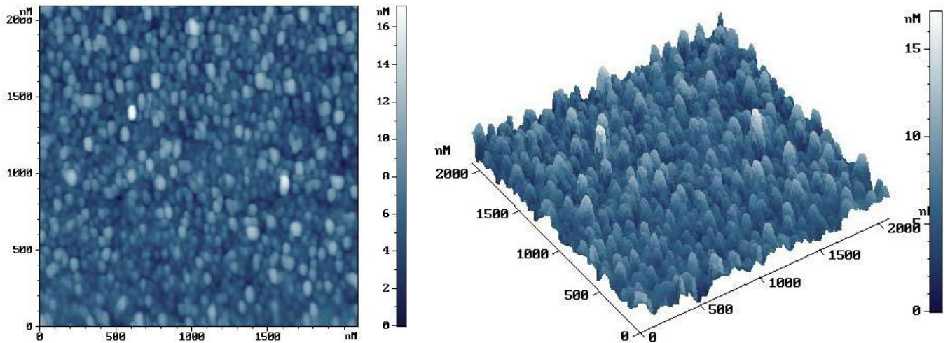
Рисунок 4.19 – 2D (слева) и 3D (справа) изображения АСМ исследования рельефа на поверхности нитрида кремния в периферийной области (в зоне лазерного расплава) пятна облучения ArF-лазером ( \lambda = 193 нм, 20 импульсов; 4.5 \text{ Дж/см}^2 , частота 10 Гц)
